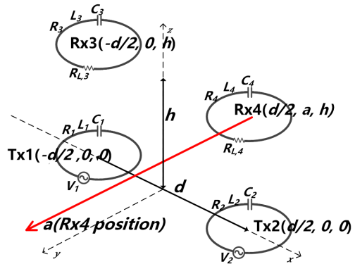
그림 2. 2x2 MIMO 무선전력전송 시스템 Fig. 2. 2x2 MIMO wireless power transmission system.
