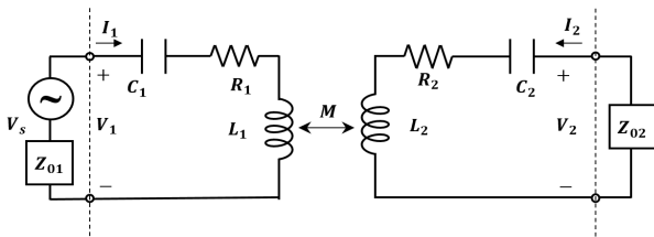
그림 1. 자유공간 자기공진 무선전력전송 시스템 Fig. 1. Magnetic resonance WPT system in free space.
